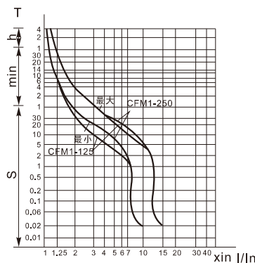
图1 CFM1-(100)125、(225) 250型断路器保护特性曲线
