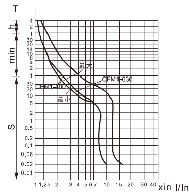
图2 CFM1-400、630、800 型断路器保护特性曲线
